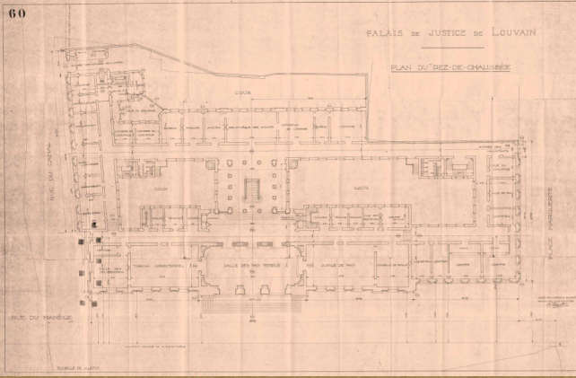
Plan met ontwerp van de gelijkvloerse verdieping van het Leuvens gerechtshofgebouw, Oscar Francotte, 30 juli 1922. Collectie Rijksarchief Leuven.
