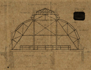
Plan met dwarsdoorsnede van de koepel van het Leuvens gerechtshofgebouw, Oscar Francotte, 31 maart 1925. Collectie Rijksarchief Leuven.
